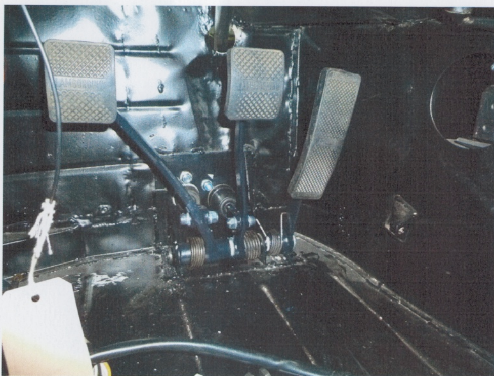
Einbau und anpassen der Hydraulikzylinder
